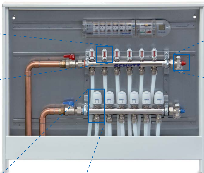
Collettore della mandata DN 25 con misuratore di portata ruotabile incorporato.
